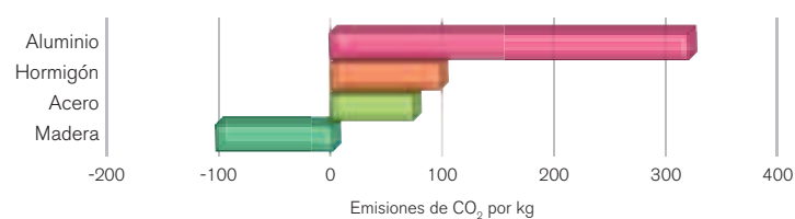
Vigas: producción de CO 2
